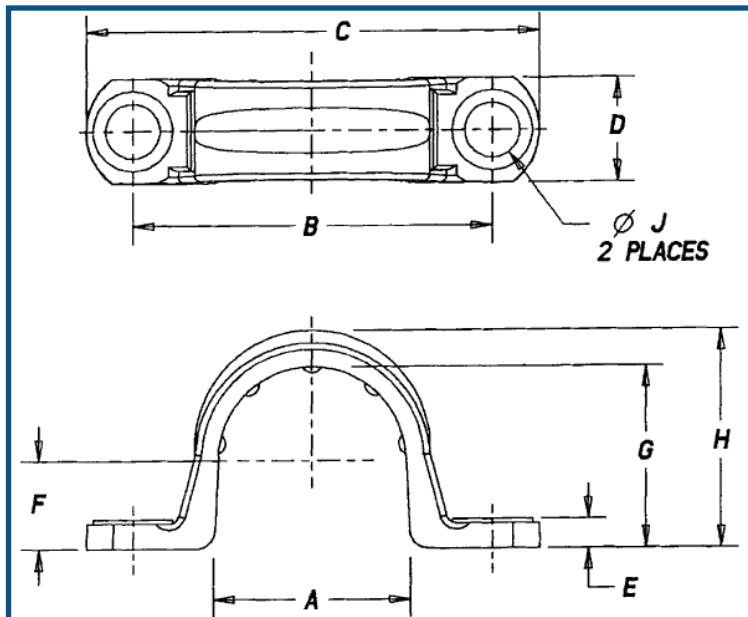
CONDUIT CLAMP
